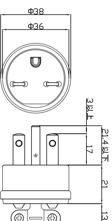
単相200Vプラグ形状 (接地極付 15A 250V)
