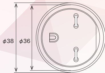
単相200Vプラグ形状図
