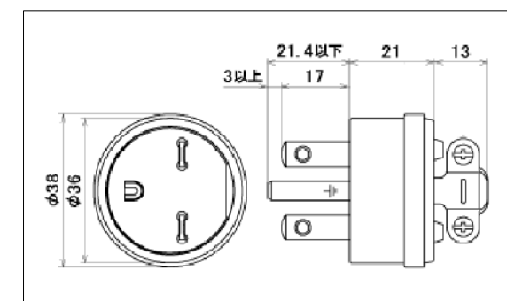
単相200Vプラグ形状 (接地極付 15A 250V)
